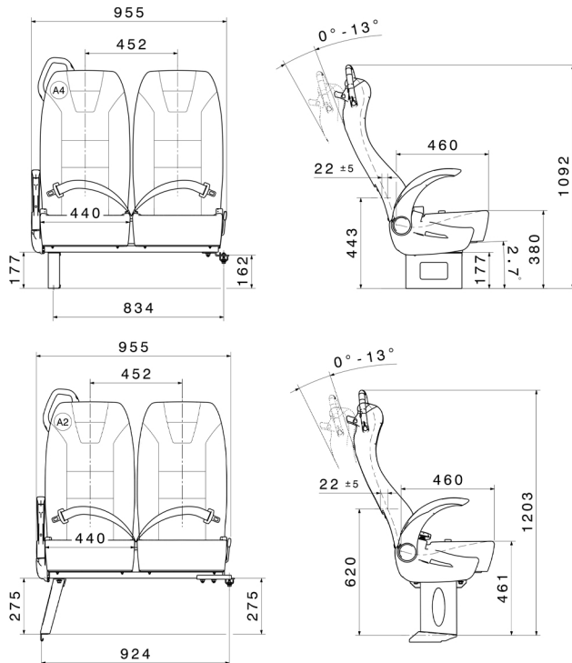
Koridor Tarafı Yukarı Katlanır Kolçak Aisle-side Foldable (Up) Korridor Seite Klappbar Nach Oben Lado Pasillo - Plegable (Arriba)
